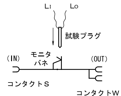
MT20-TS1-8 切分け端子板
