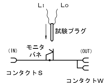
MT20-TS1 切分け端子板
